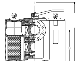
Sivukuva kierre-mallit
