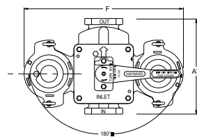
Yläkuva kierre-mallit
